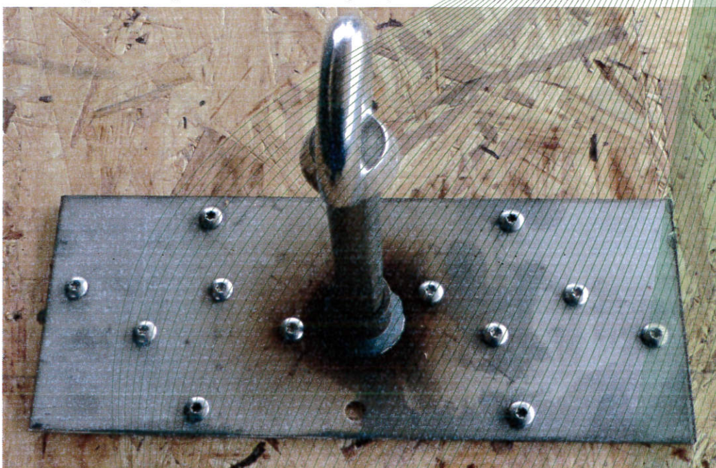
Bild 1: Beispiel der Anschlageinrichtung, Typ: Primo 7 OSB
